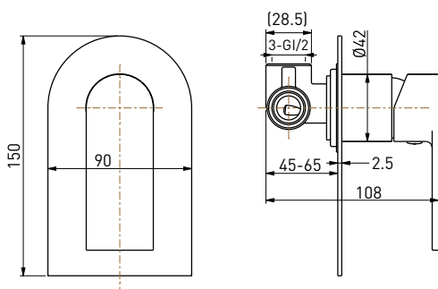
Mixer FO-M
