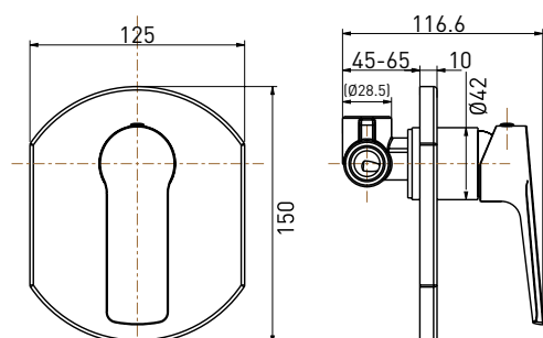
Mixer SP-M
